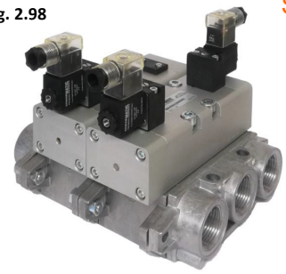
ISO 3 VALFLER ISO 3 SERIE VALVES
